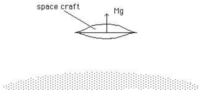
34. ábra. Ugyanez a helyzet az iker-Világegyetemből tekintve. A Föld itt láthatatlan, a taszító ereje azonban jelen van.
