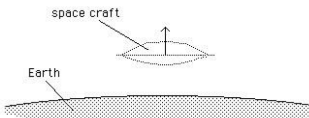
33. ábra. Az űrhajó eltűnik az iker-Világegyetembe. A földi megfigyelő számára láthatatlanná válik, és eltávolodik a bolygótól annak negatív mg ereje miatt.
