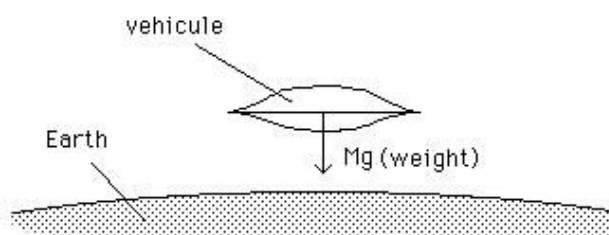
32. ábra. Az űrhajó a mi Világegyetemünkben tartózkodik. Hat rá a súlya, mg . Ahol m a tömege, g a gravitációs gyorsulás.
